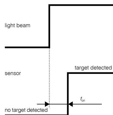
Fig. 47: Output turn-on time
