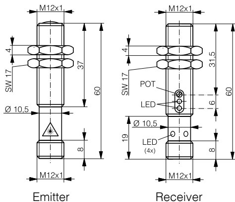
Emitter
